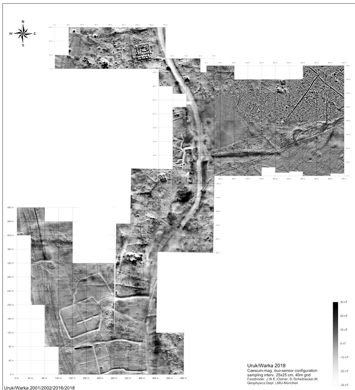
Рис. 4. Магнитограмма участков обзора 1, 3 и 4
