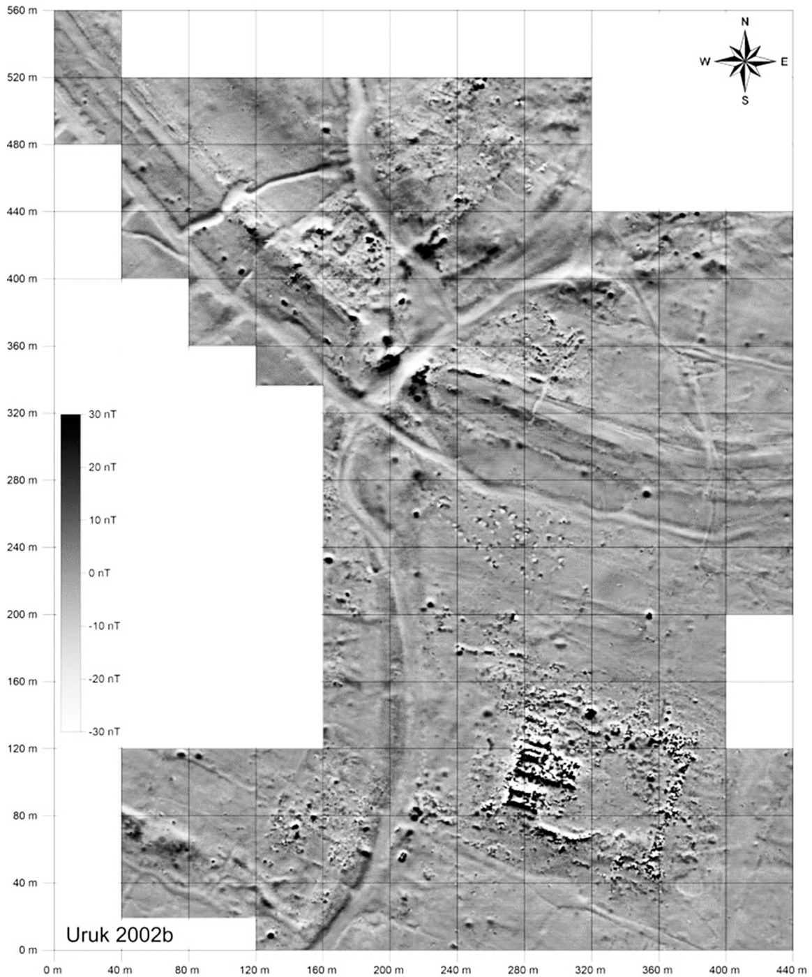
Рис. 5. Магнитограмма зоны обзора 2 Fig. 5. Magnetogram of the viewing area 2
