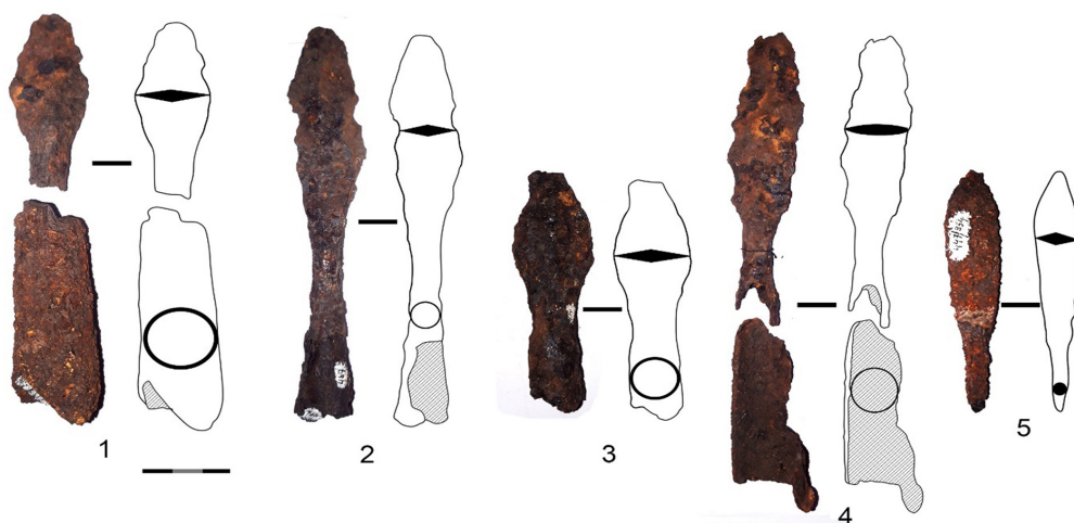
Рис. 3.* Наконечники копий Кушулевского III могильника: 1 – п. № 18; 2 – п. № 96; 3 – п. № 175; 4 – п. № 189; 5 – п. № 59
